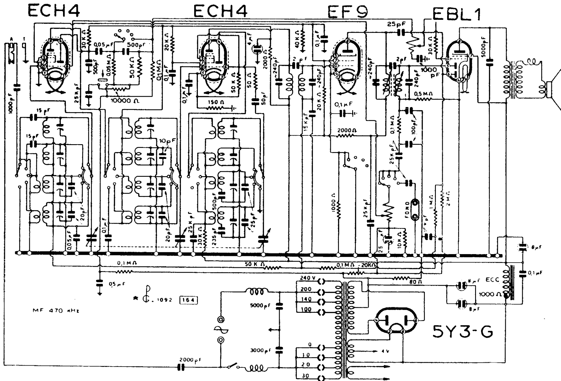
F.I.M.I. - MOD. PHONOLA « 571 »
